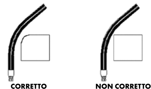
FIG. 1 - PREVENZIONE DANNI ESTERNI SUL TUBO
