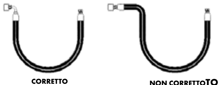
FIG. 3 – CURVE ED ADATTATORI
